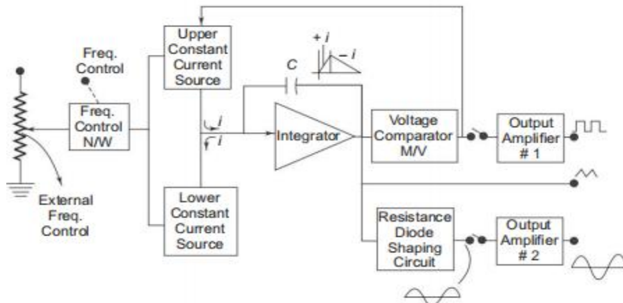
Fig. 8.5 Function generator
